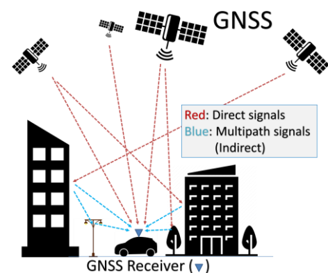
Fig. 1. GNSS multipath error
